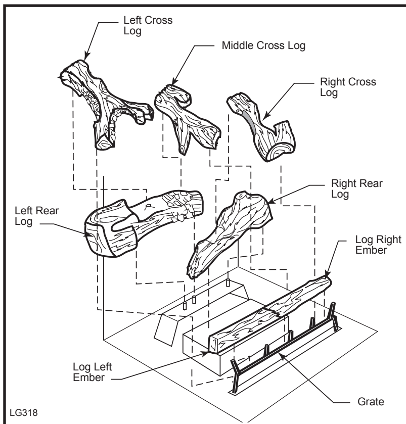
Fig. 14 ODGSR42A log placement.
